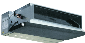
Рис. 1. Канальный внутренний блок PEAD-RP125EA
