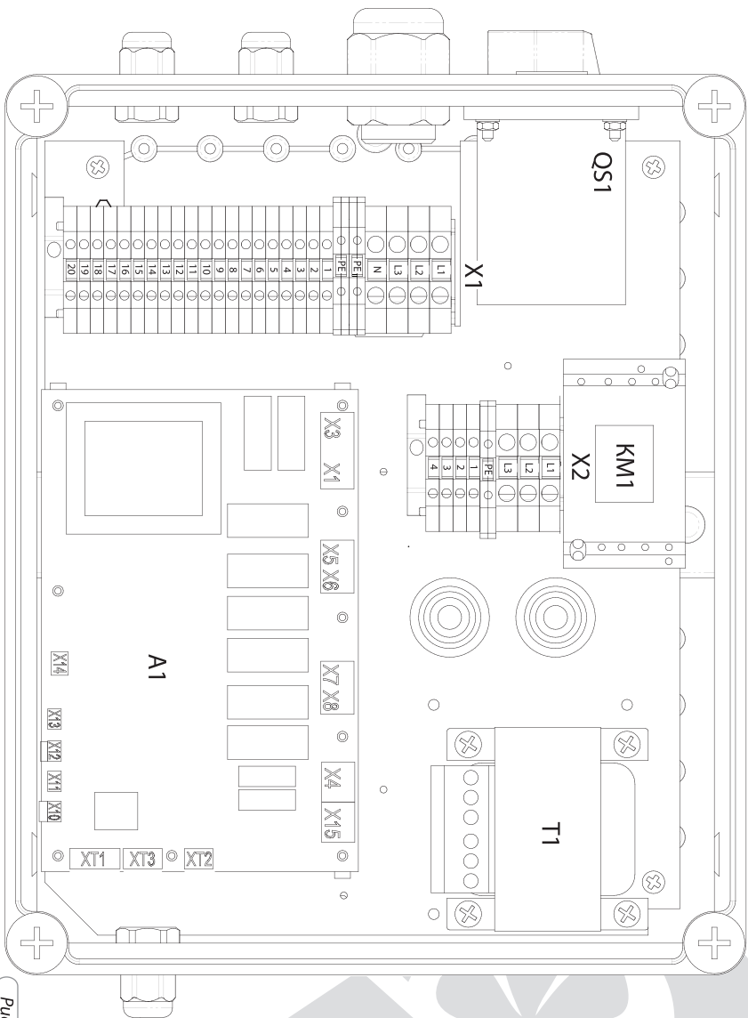
Блок управления для трехфазной сети 400 В/ 50 Гц Крышка условно не показана
